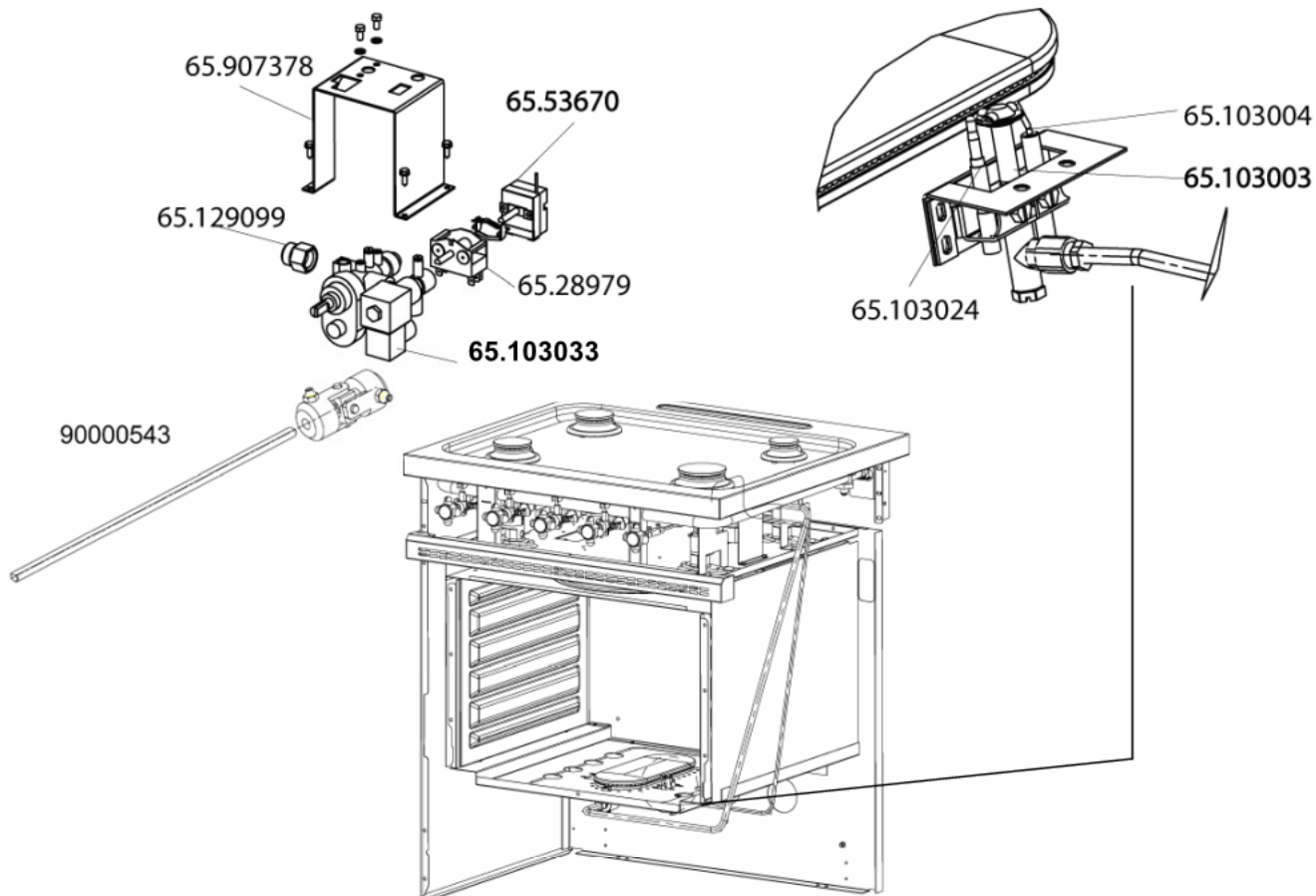
Détail A:
