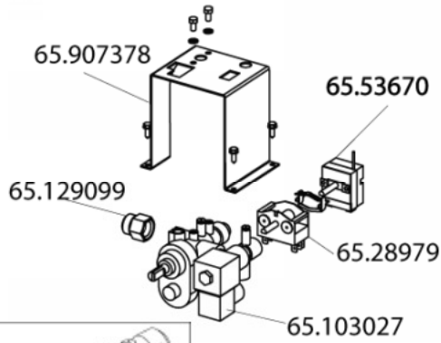
Détail A :
